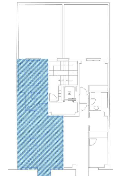
Planta Quinta y Atico. E: 1/200
