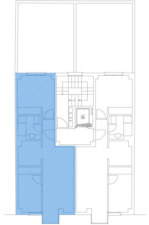
Planta Tipo. E: 1/200
